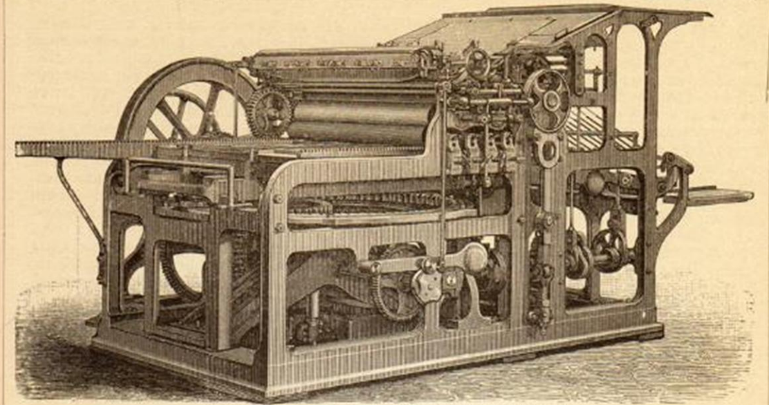
1. Простая скоропечатная машина (Кенигъ и Бауеръ).
